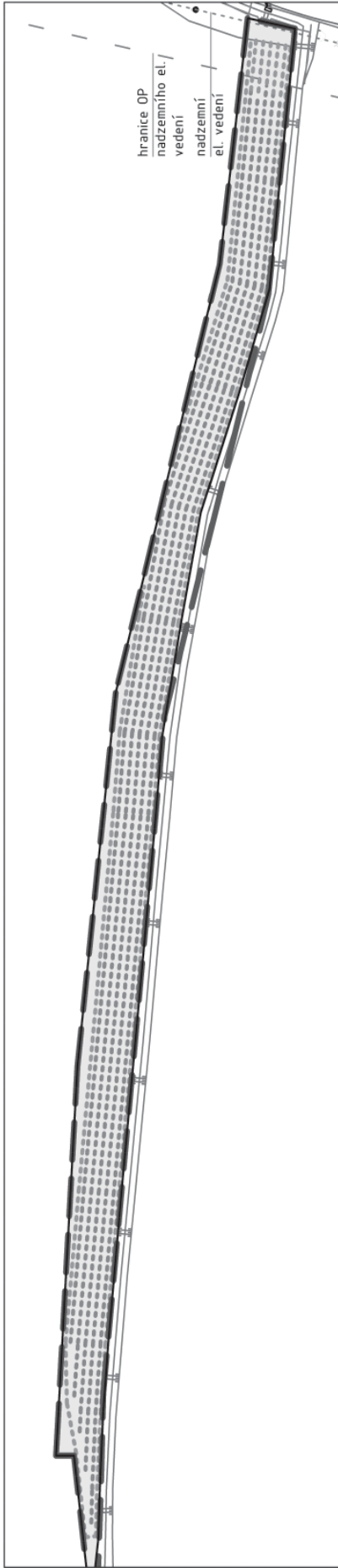
NÁVRH VÝSADBY VĚTROLAMU, 1:750
